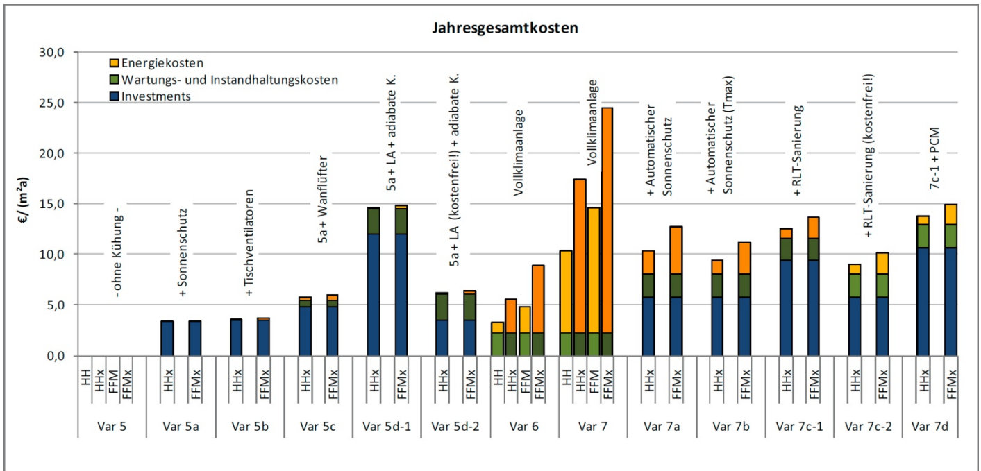
Abbildung 3: Darstellung der Jahresgesamtkosten für die untersuchten Optimierungsvarianten der Bürogebäude 5 und 7.
