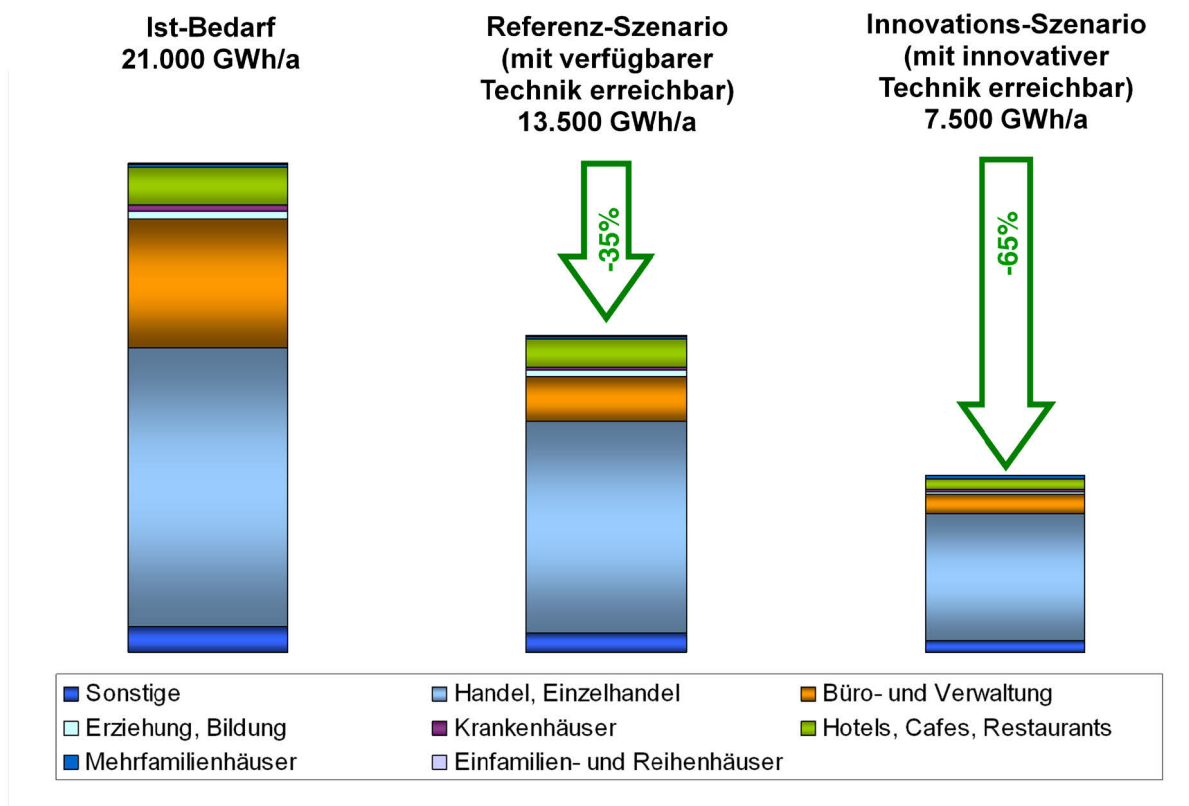
Abbildung 6: Beim Szenario „Umsetzung des technischen Potenzials“ wird davon ausgegangen, dass sofort die im Jahr 2009 verfügbaren Maßnahmen und Effizienztechniken zur Verringerung des Endenergiebedarfs zur Kühlung umgesetzt werden. Dadurch ergeben sich beim Referenzszenario Einsparungen von etwa 33 % und beim Innovationsszenario von 64 %. Wie auch deutlich zu sehen ist, besteht bei den Bürogebäuden das größte Einsparpotenzial von etwa 5,5 GWh/a (Basis) auf etwa 2 GWh/a beim Referenz- bzw. 1 GWh/a beim Innovationsszenario.
