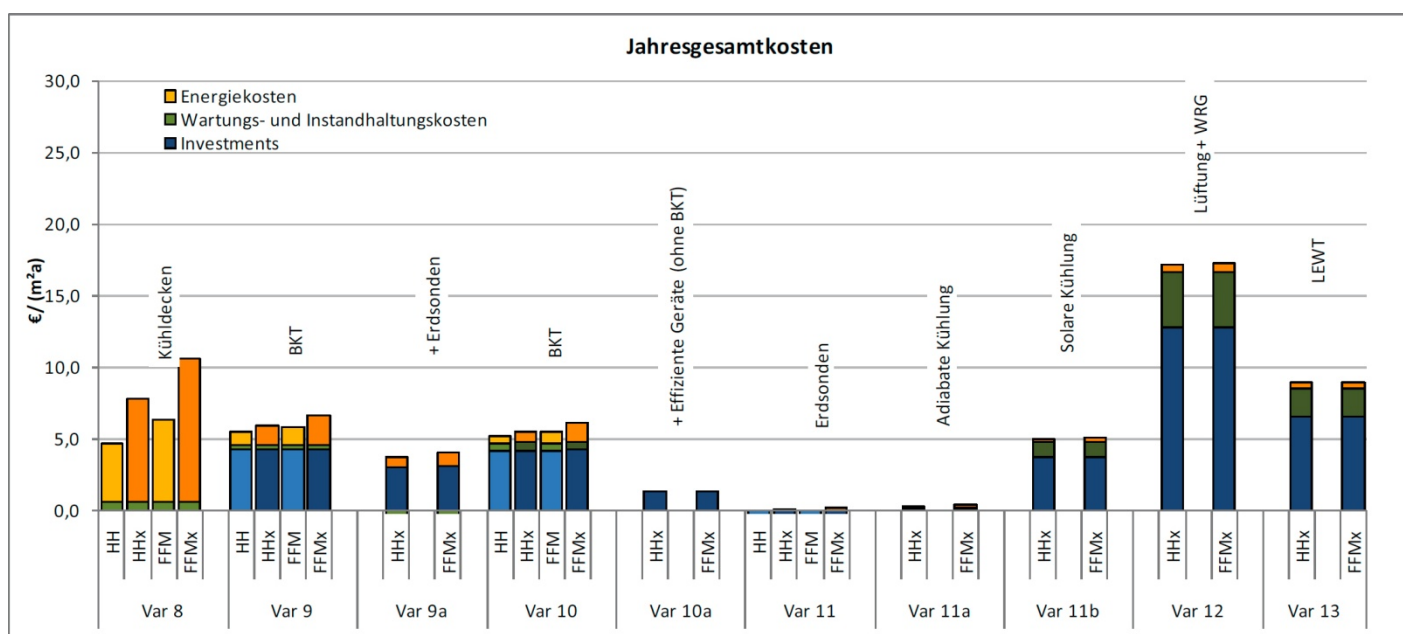
Abbildung 4: Darstellung der Jahresgesamtkosten für die untersuchten Optimierungsvarianten der Bürogebäude 8 bis 11.
