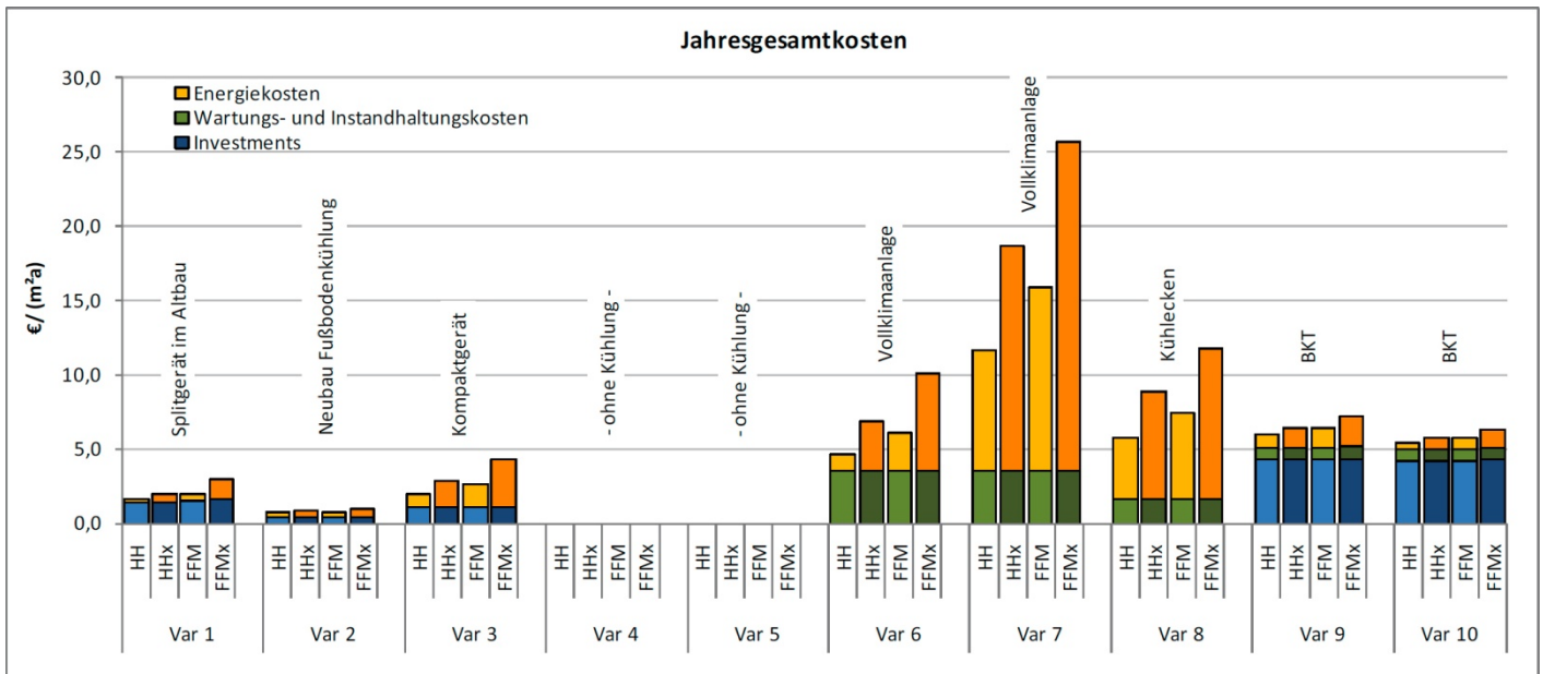
Abbildung 2: Darstellung der Jahresgesamtkosten für die untersuchten vier Varianten der Wohngebäude und die sechs Varianten der Bürogebäude
