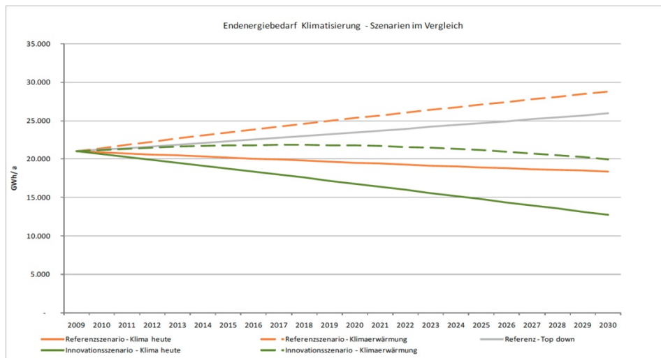
Abbildung 5: Die Ergebnisse zum Endenergiebedarf zur Gebäudekühlung im Jahr 2030 bei den verschiedenen Szenarien unter Berücksichtigung von „keiner“ und einer Klimaerwärmung um 2 K.
