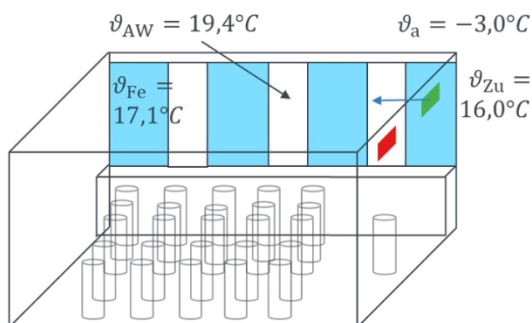
Bild 9-1: Randbedingungen der Strömungssimulation im Winter- und Sommerfall
