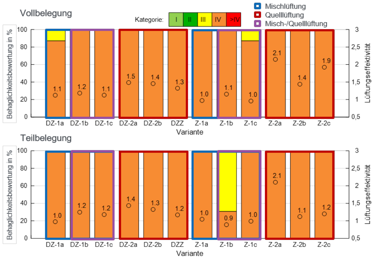
Bild 9-4: Gesamtauswertung der Luftführungskonzepte für Frontalunterricht im Sommerfall
