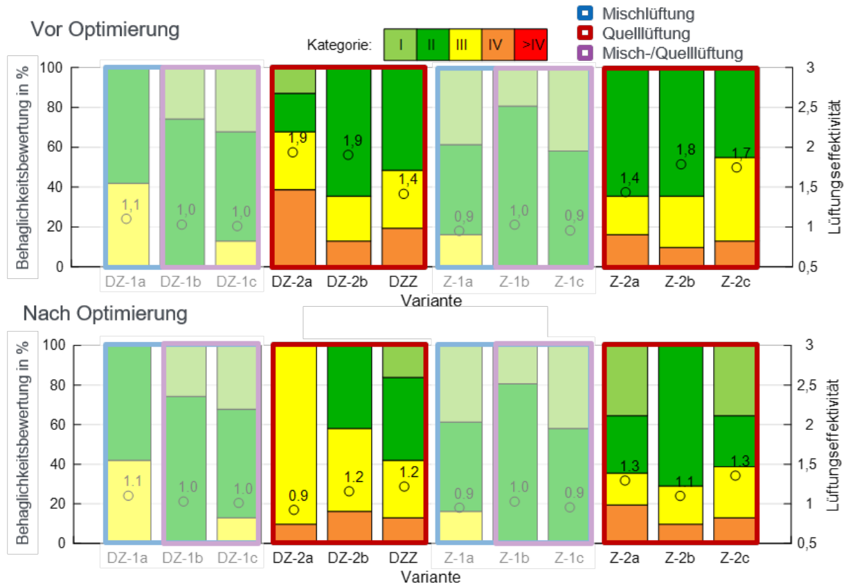
Bild 9-5: Gesamtauswertung der Luftführungskonzepte für Frontalunterricht im Winterfall, Angepasster Luftwechsel nach Lüftungseffektivität
